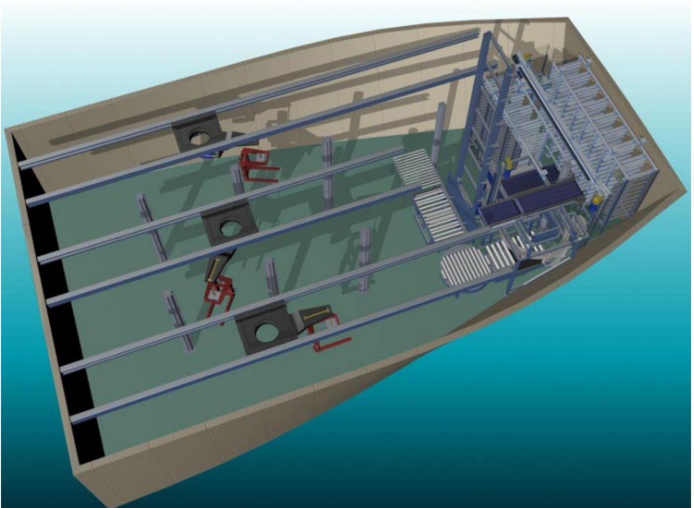
Lasterom med mellomlager, palleterer og transportsystemer
