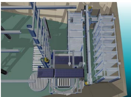
Mellomlager og palleterer
